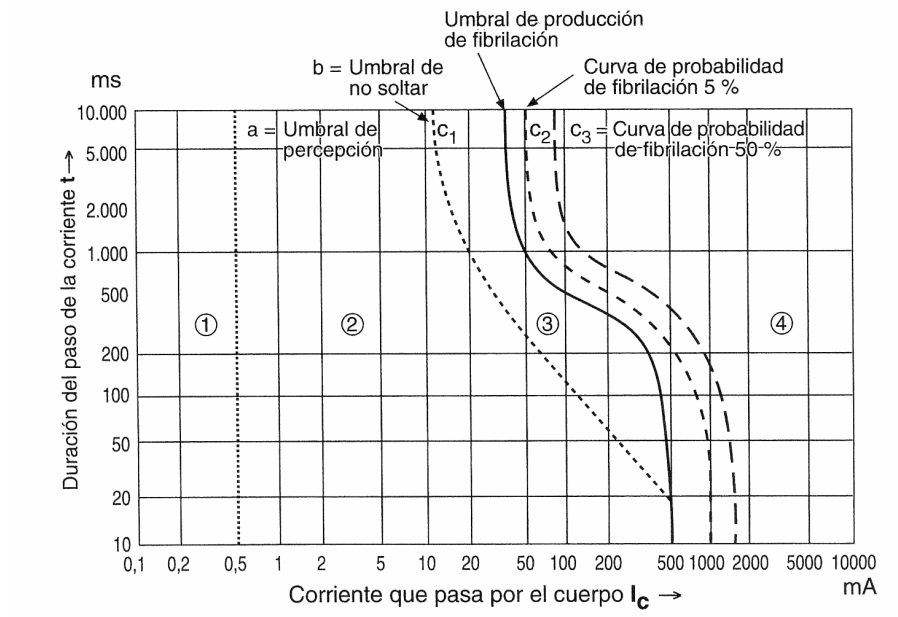
FIGURA 9.1: Efecto de la corriente que circula por el cuerpo humano según su intensidad y tiempo de duración [84, 85].
