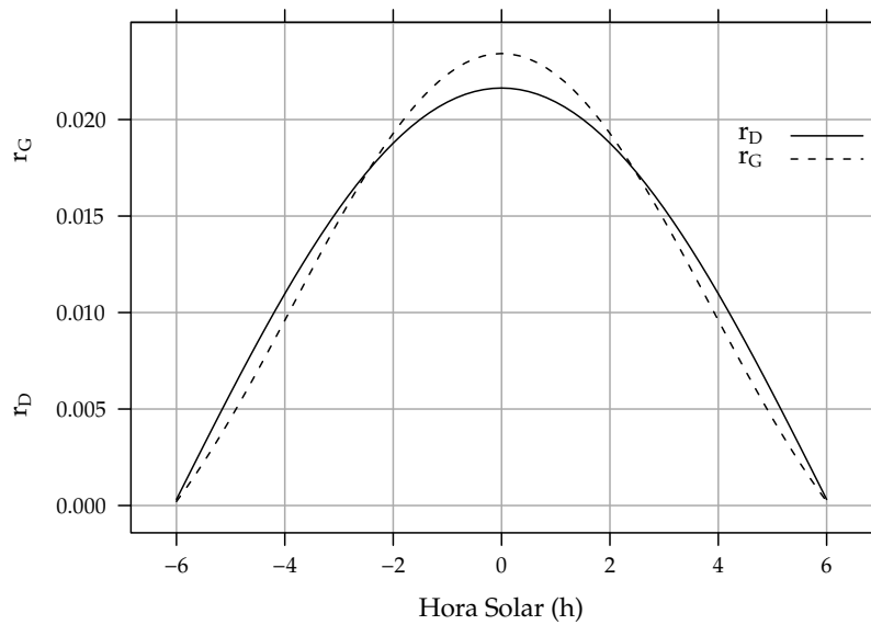
FIGURA 3.4: Perfil de irradiancia difusa y global obtenido a partir del generador empírico de [31] para valores de irradiancia tomadas cada 10 minutos.
