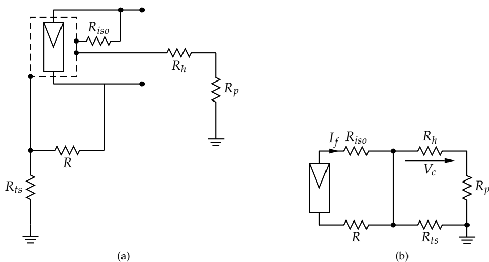
FIGURA 9.6: Esquema eléctrico de contacto indirecto en un sistema fotovoltaico con esquema de conexión a tierra TN.
