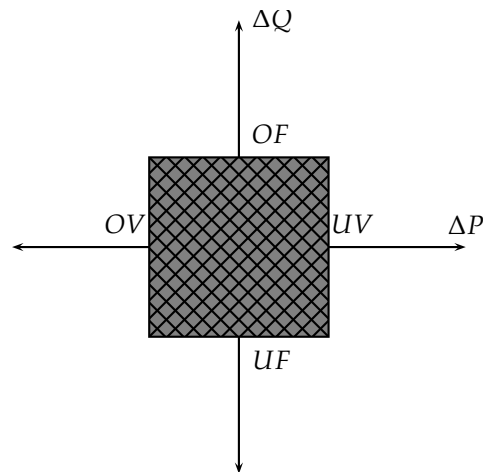
FIGURA 6.6: Zona de no detección en modo isla. Cualquier combinación de potencia activa y reactiva de red antes de la desconexión que se encuentre dentro de esa región implica que el inversor continuaría funcionando en modo isla durante un tiempo.
