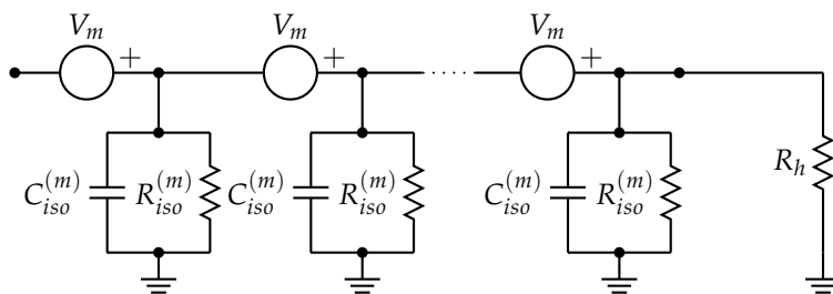
FIGURA 9.4: Capacidad distribuida en un generador fotovoltaico con esquema de conexión a tierra TT.
